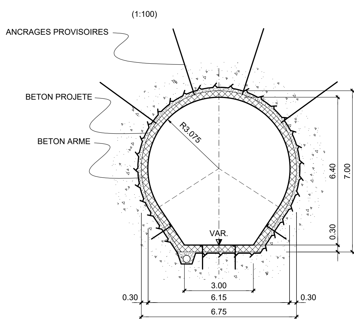
COUPE TYPE PUIITS INCLINE (B-B)
