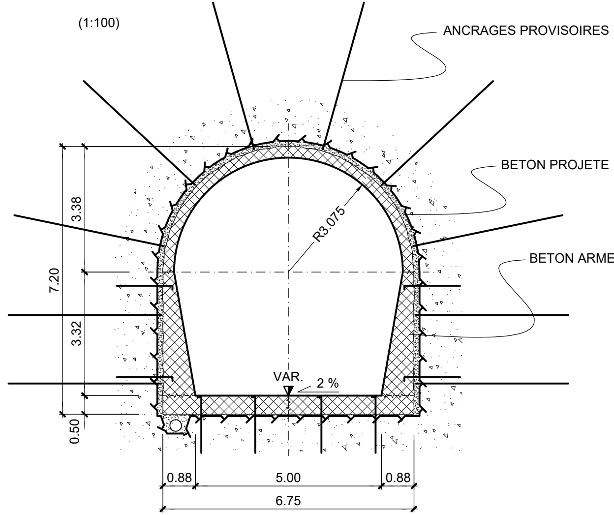
COUPE TYPE GALERIE DE DECHARGE (A-A)
