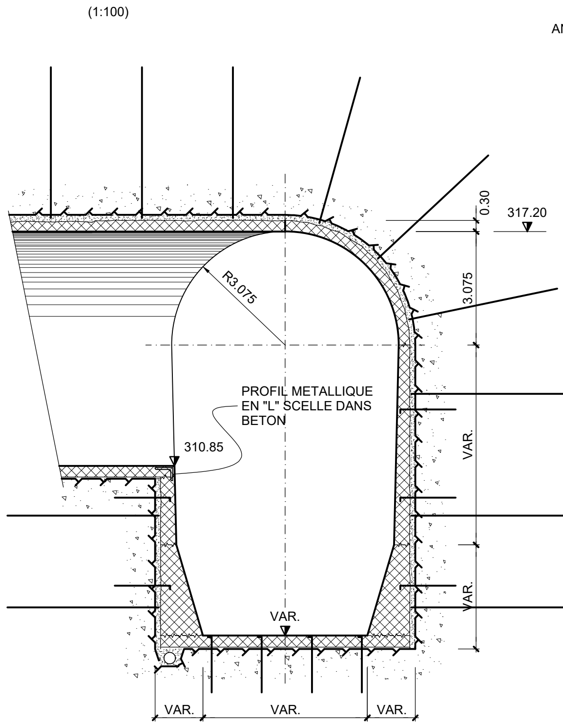
COUPE TYPE INTERSECTION CANAL DE DECHARGE ET PUIITS INCLINE (C-C)
